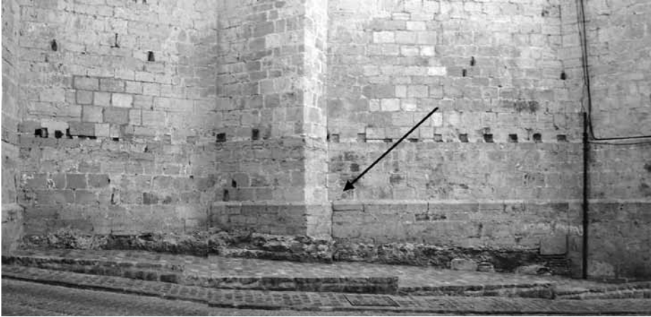
Basaments de l'absis on es veu el llit de morter on descansa la sillera
