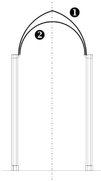
Esquema de les voltes: 1- Volta gòtica amb nervadures i closca de rajoles verticals 2- Volta barroca amb closca de rajoles horitzontals
