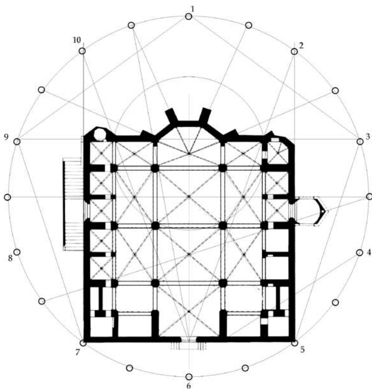
Traçat geomètric de la planta de l'església de Santa Maria de Sagunt
